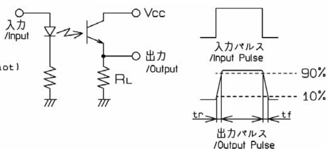
図2 応答速度
