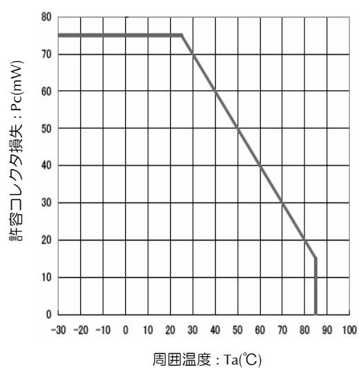
周囲温度－コレクタ損失 特性
