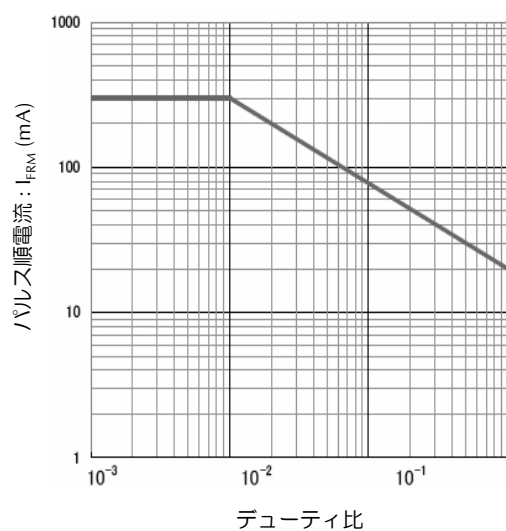
デューティ比－パルス順電流 特性
