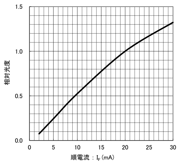
順電流 vs. 相对光度 特性
