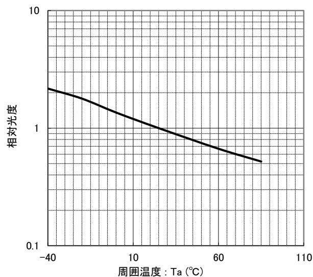
周囲温度 vs. 相对光度 特性
