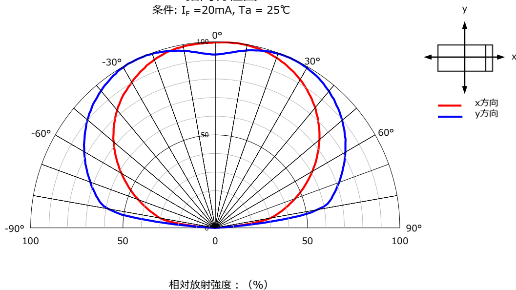
指向特性図
