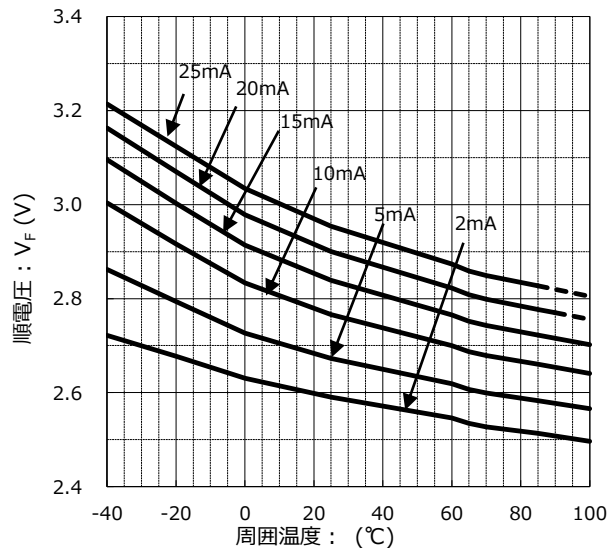
周囲温度 vs. 順電圧 特性 条件: I_F = 2 \sim 25\text{mA}
