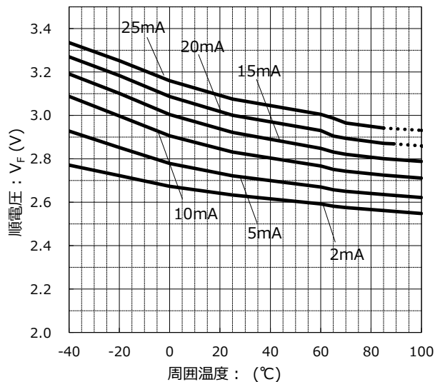
周囲温度 vs. 順電圧 特性 条件 : I_F = 2 \sim 25\text{mA}
