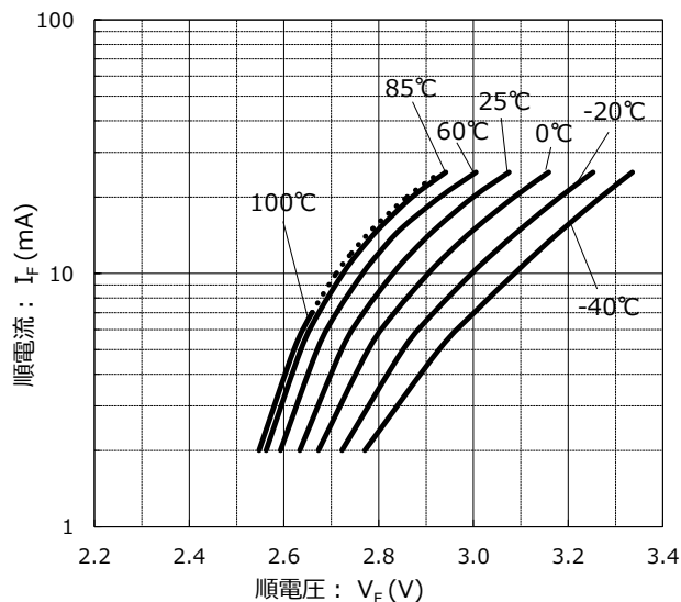
順電圧 vs. 順電流 特性 条件 : T_a = -40 \sim 100^\circ\text{C}
