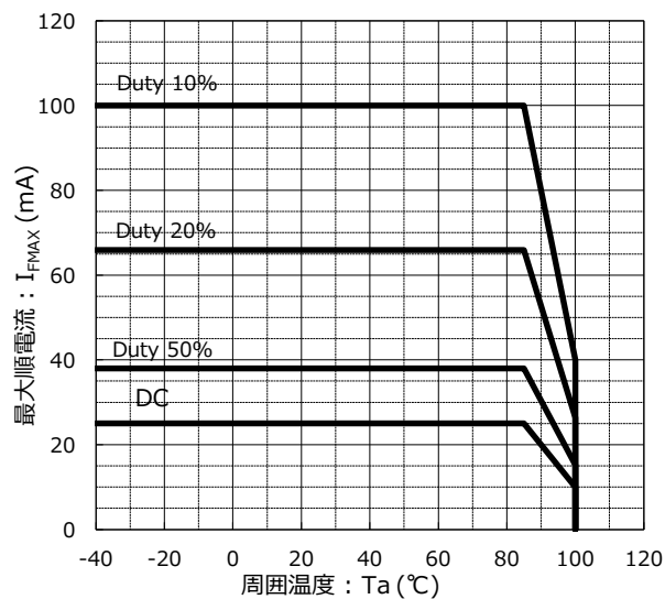
順電流低減定格 繰り返し周波数 : f \geq 100\text{Hz}
