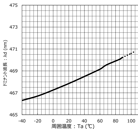
周囲温度 vs. ドミナント波長 特性 条件 : I_F = 20\text{mA}
