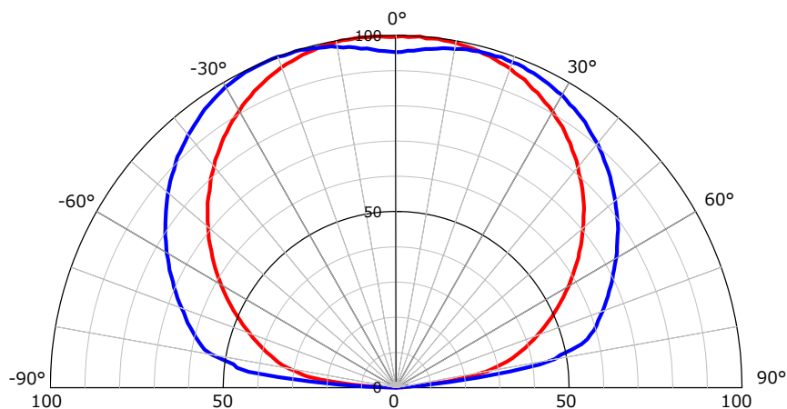
指向特性図
