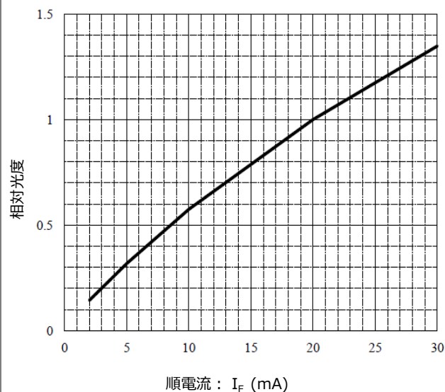
順電流 vs. 相対光度 特性
