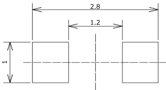
対称パッド
