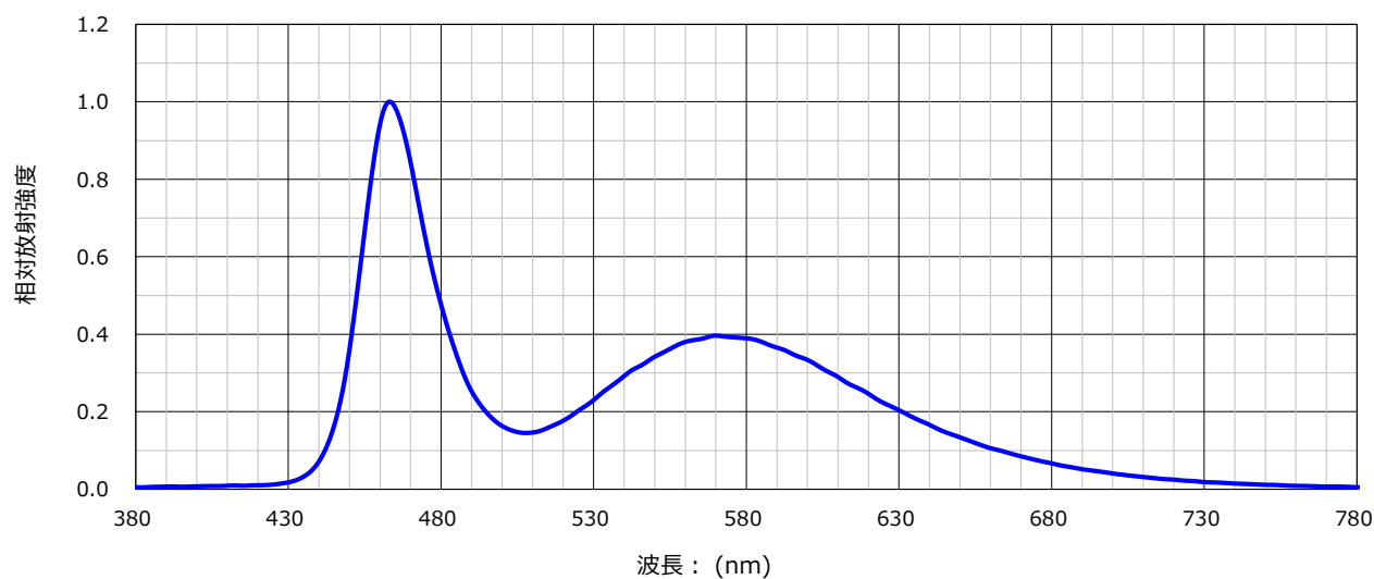
スペクトル分布特性 条件: I_F=10\text{mA} , T_a=25^\circ\text{C}
