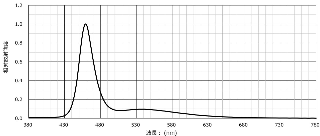
スペクトル分布特性 条件: I_F=10\text{mA} , T_a=25^\circ\text{C}
