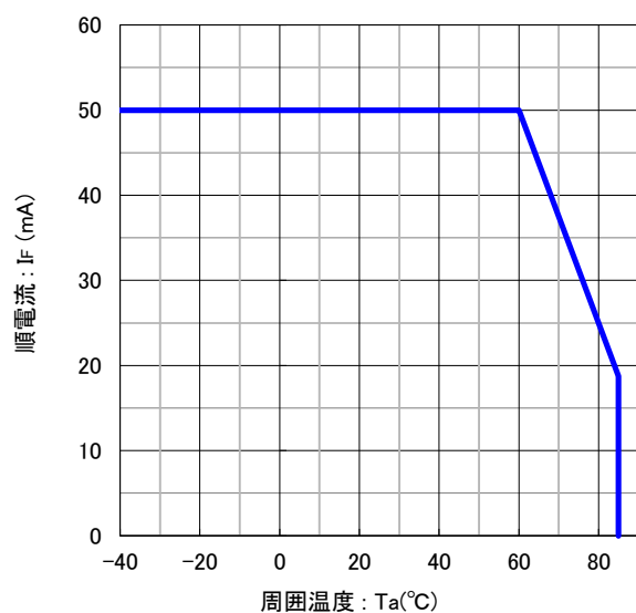
周囲温度 vs. 順電流 特性
