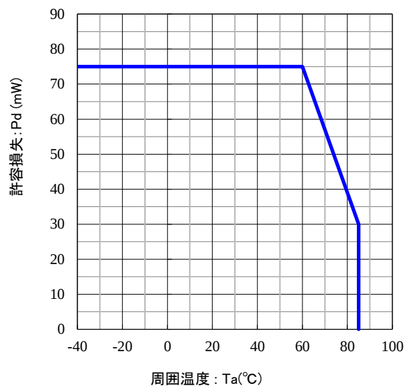
周囲温度 vs. 許容損失 特性
