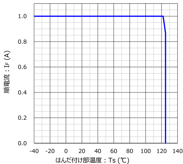
順電流定格
