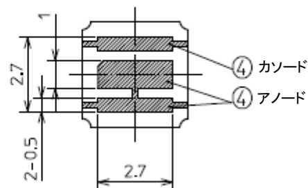
裏面図
