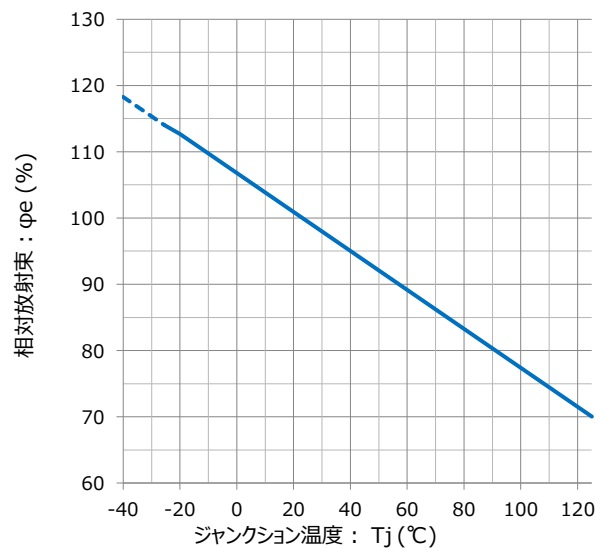
ジャンクション温度 vs. 放射束 特性
