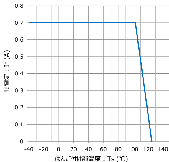
順電流定格
