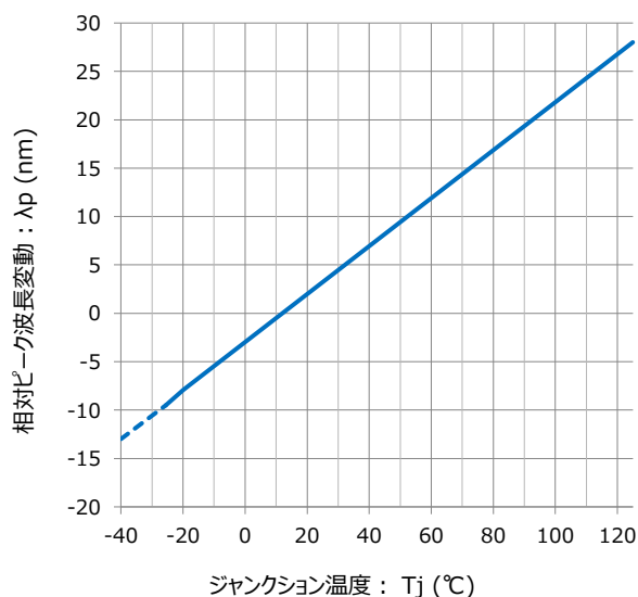
ジャンクション温度 vs. ピーク発光波長 特性
