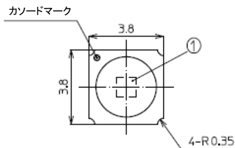
上面図
