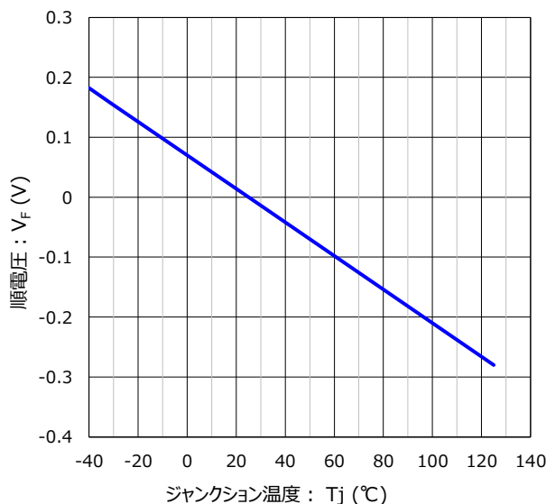
ジャンクション温度 vs. 順電圧 特性 条件 : I_F = 1\text{A}
