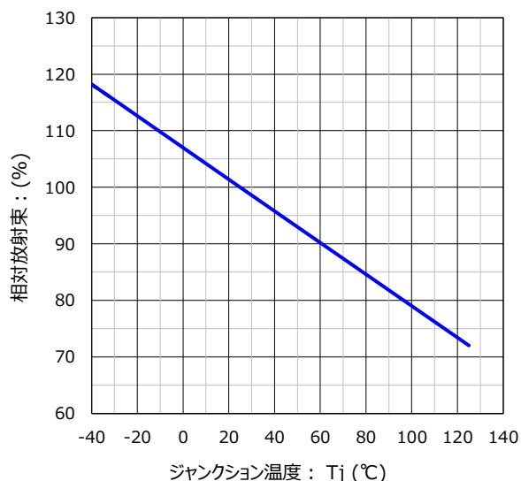
ジャンクション温度 vs. 相対放射束 特性 条件 : I_F = 1\text{A}
