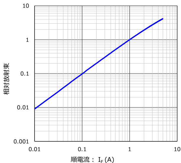
順電流 vs. 相対放射束 特性 条件 : T_a = 25^\circ\text{C} , シングルパルス ( t_w=100\mu\text{s} )
