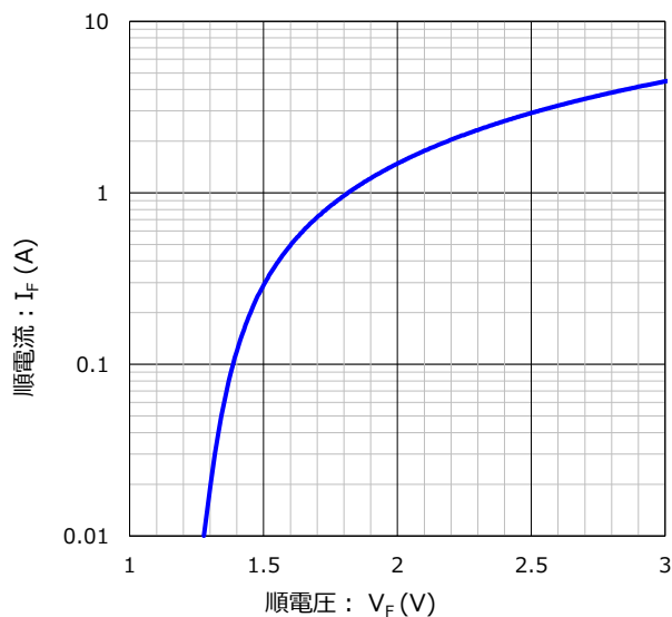
順電圧 vs. 順電流 特性 条件 : T_a = 25^\circ\text{C} , シングルパルス ( t_w=100\mu\text{s} )
