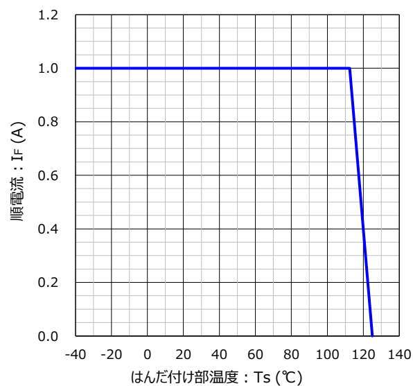
順電流定格
