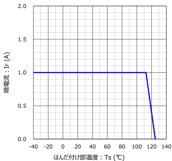
順電流定格
