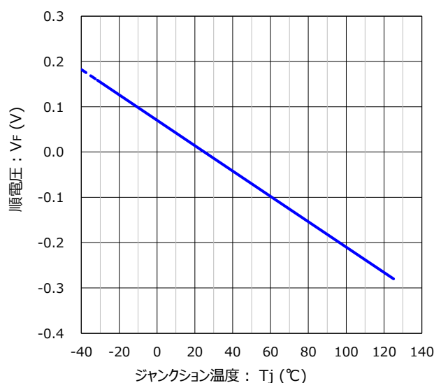
ジャンクション温度 vs. 順電圧 特性
