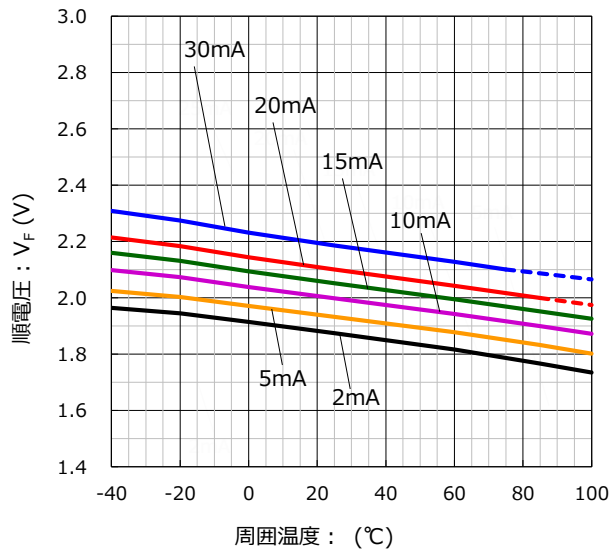
周囲温度 vs. 順電圧 特性 条件 : I_F = 2 \sim 30\text{mA}
