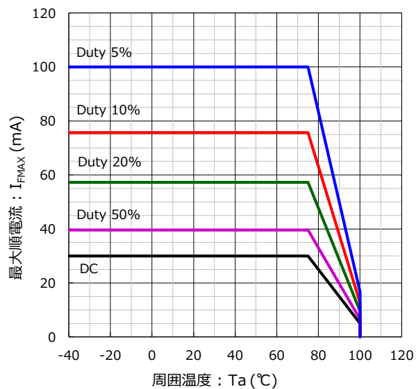
順電流低減定格 繰り返し周波数 : f \geq 50\text{Hz}
