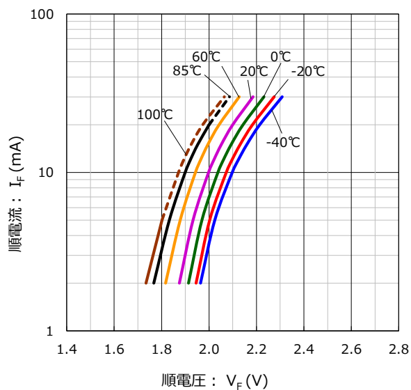
順電圧 vs. 順電流 特性 条件 : T_a = -40 \sim 100^\circ\text{C}
