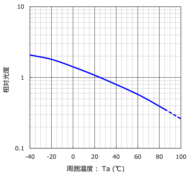
周囲温度 vs. 相対光度 特性 条件 : I_F = 20\text{mA}
