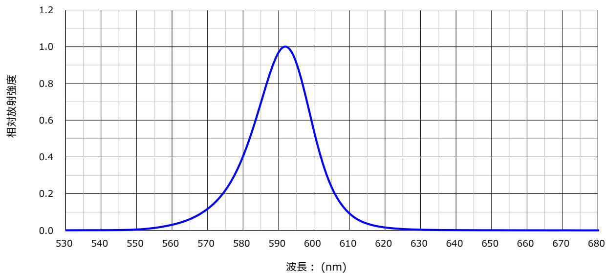
スペクトル分布特性 条件: I_F = 20\text{mA} , T_a = 25^\circ\text{C}
