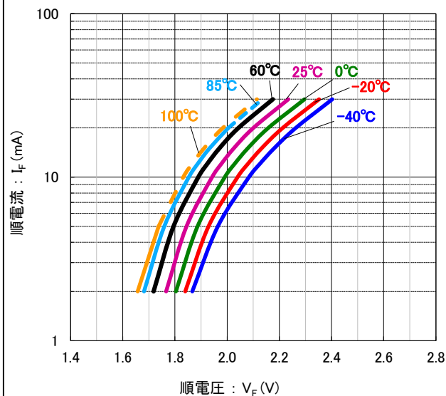
順電圧 vs. 順電流 特性
