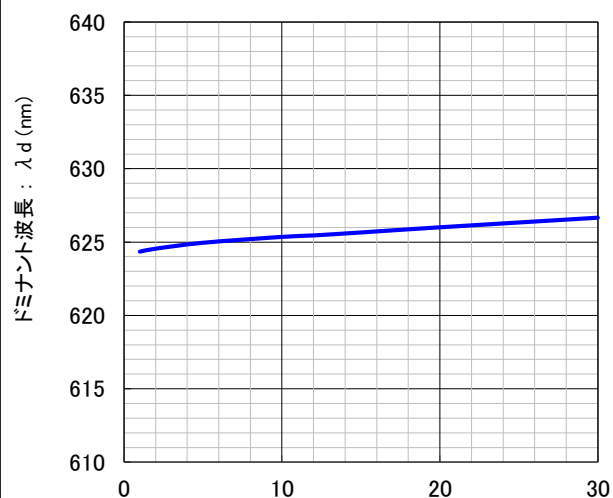
順電流ードミナント波長 特性
