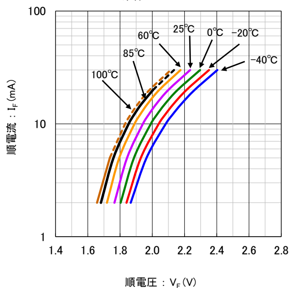
順電圧－順電流 特性
