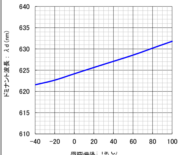
周囲温度ードミナント波長 特性
