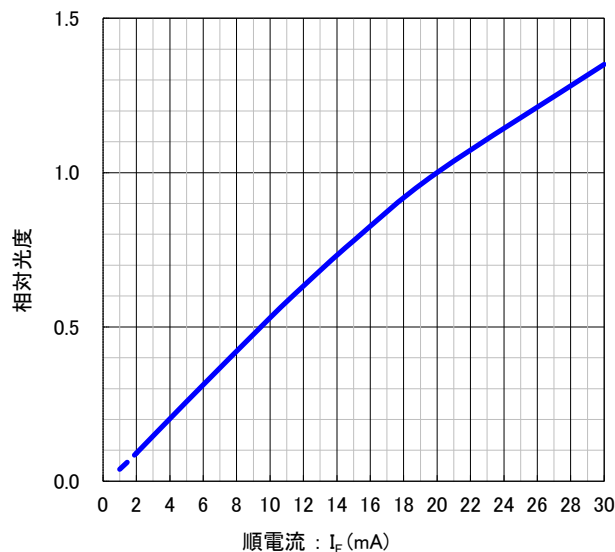
順電流 vs. 相对光度 特性
