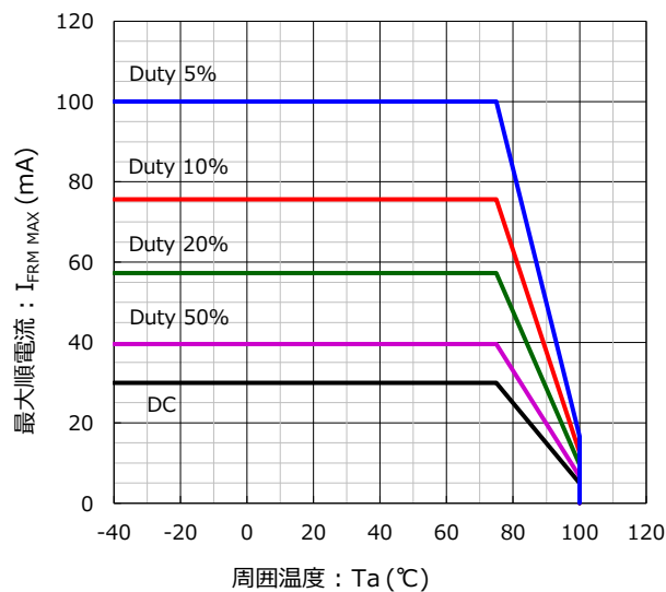
順電流低減定格 繰り返し周波数 : f \geq 50\text{Hz}
