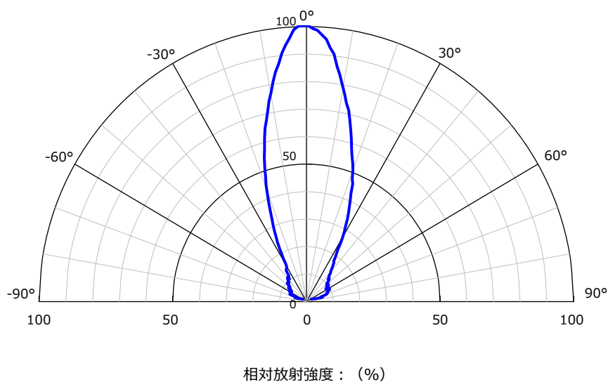
指向特性図 条件: I_F = 20\text{mA} , T_a = 25^\circ\text{C}
