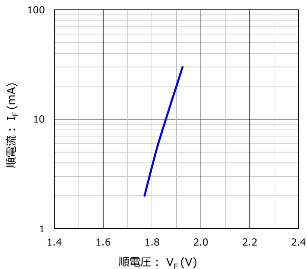
順電圧 vs. 順電流 特性 条件 : T_a = 25^\circ\text{C}
