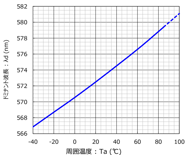
周囲温度 vs. ドミナント波長 特性 条件 : I_F = 20\text{mA}
