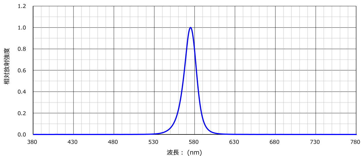
スペクトル分布特性 条件: I_F = 20\text{mA} , T_a = 25^\circ\text{C}
