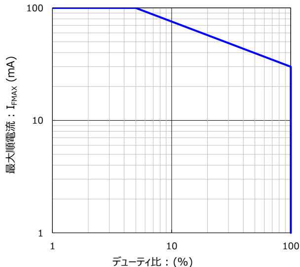
ダイナミック点灯定格 パルス幅 : t_w \leq 1\text{ms}
