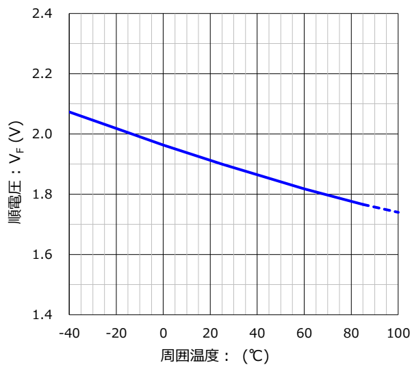
周囲温度 vs. 順電圧 特性 条件 : I_F = 20\text{mA}
