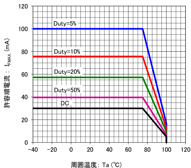
順電流低減定格
