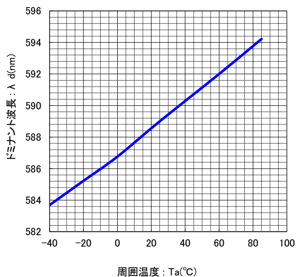
周囲温度ードミナント波長特性
