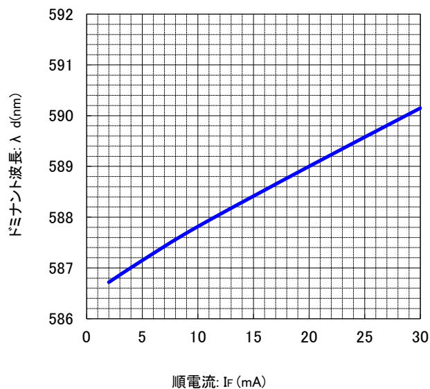
順電流ードミナント波長 特性
