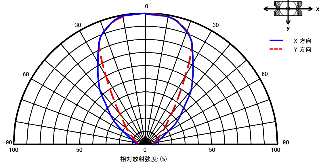
指向特性図
