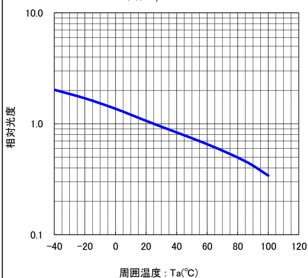
周囲温度—相対光度 特性
