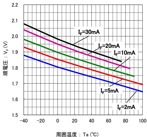
周囲温度—順電圧 特性
