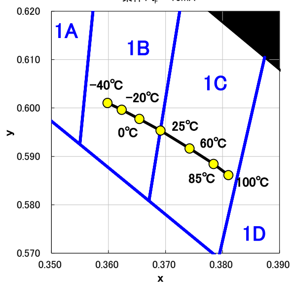
周囲温度 vs. 色度 特性
