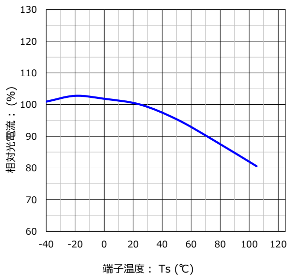
光電流温度 特性
