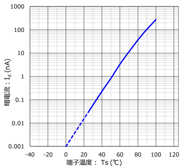
暗電流温度 特性
