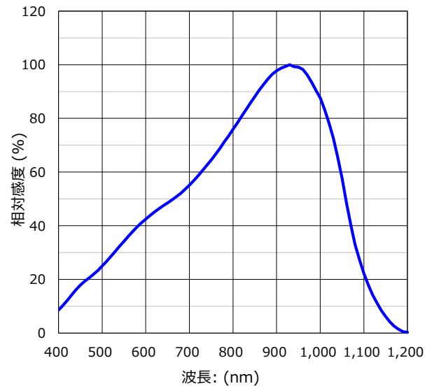
分光感度 特性
