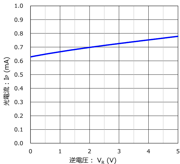
逆電圧(PD) vs. 光電流 特性
