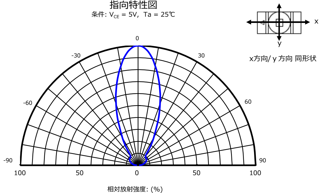
指向特性図
