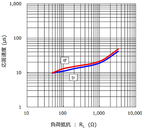
負荷抵抗 vs. 応答速度 特性
