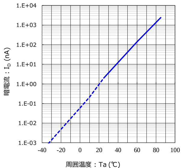
周囲温度 vs. 暗電流 特性
