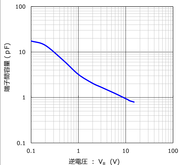
逆電圧 vs. 端子間容量 特性
