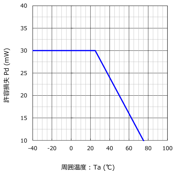
周囲温度 vs. 許容損失 特性
