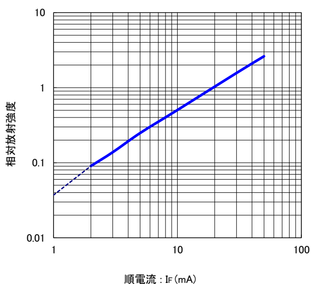
順電流 vs. 相対放射強度 特性
