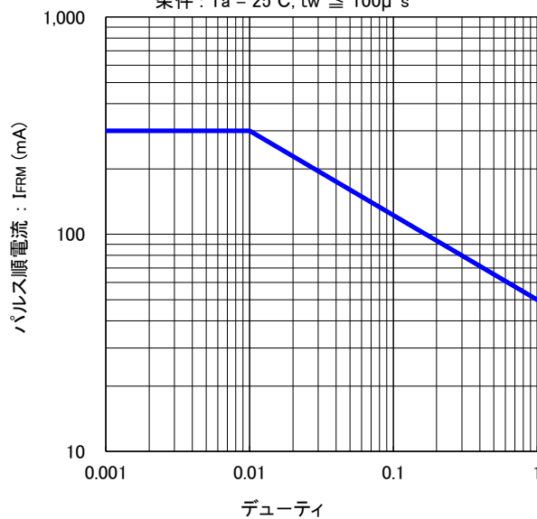
デューティ vs. パルス順電流 特性
