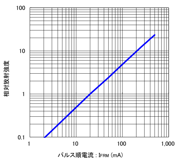
パルス順電流 vs. 相対放射強度 特性
