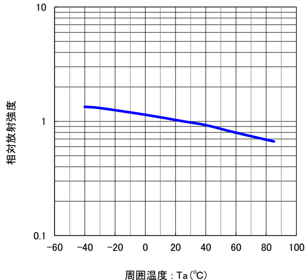
周囲温度 vs. 相対放射強度 特性
