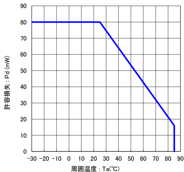
周囲温度 vs. 許容損失 特性
