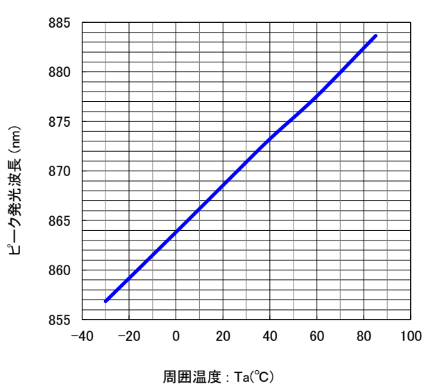
周囲温度 vs. ピーク発光波長 特性
