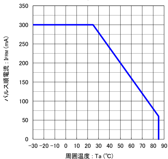
周囲温度 vs. パルス順電流 特性
