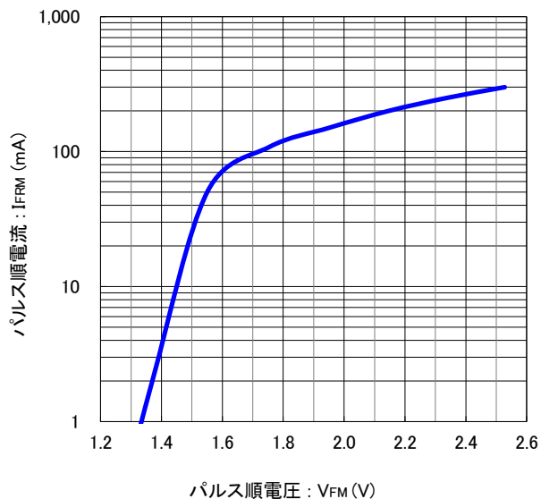
パルス順電圧 vs. パルス順電流 特性
