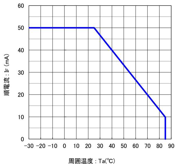
周囲温度 vs. 順電流 特性
