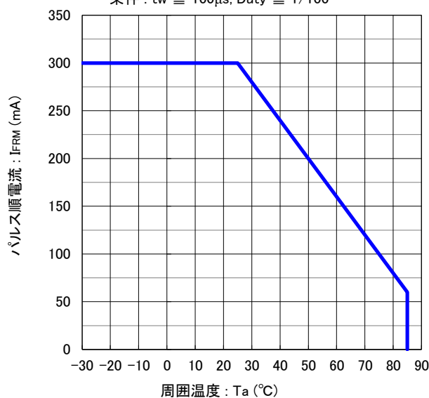
周囲温度 vs. パルス順電流 特性
