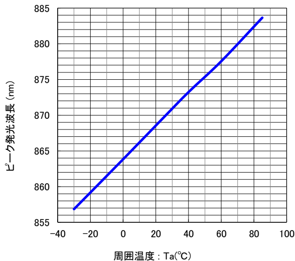
周囲温度 vs. ピーク発光波長 特性
