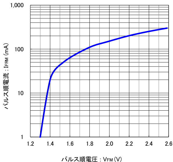
パルス順電圧 vs. パルス順電流 特性
