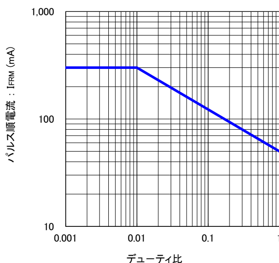
デューティ vs. パルス順電流 特性
