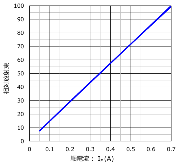
順電流 vs. 相対放射束 特性
