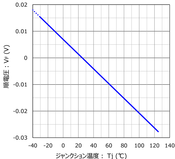
ジャンクション温度 vs. 相対順電圧 特性
