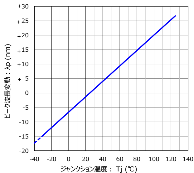
ジャンクション温度 vs. ピーク波長変動 特性
