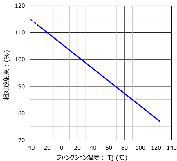
ジャンクション温度 vs. 相対放射束 特性
