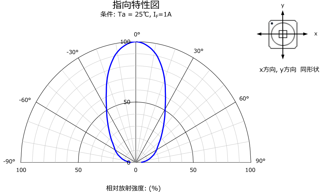
指向特性図
