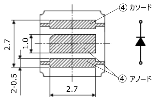
裏面図
