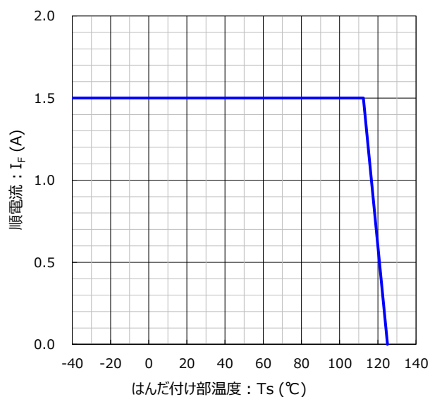
順電流定格
