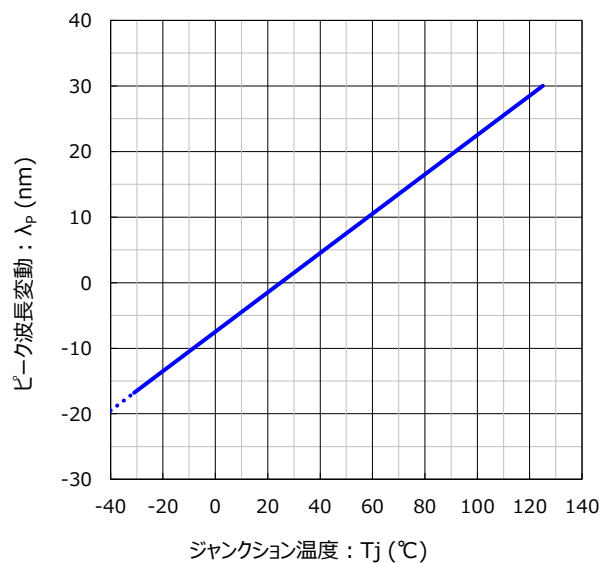
ジャンクション温度 vs. ピーク波長変動 特性
