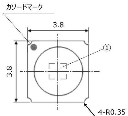
上面図
