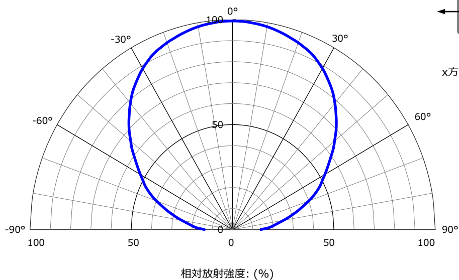
指向特性図
