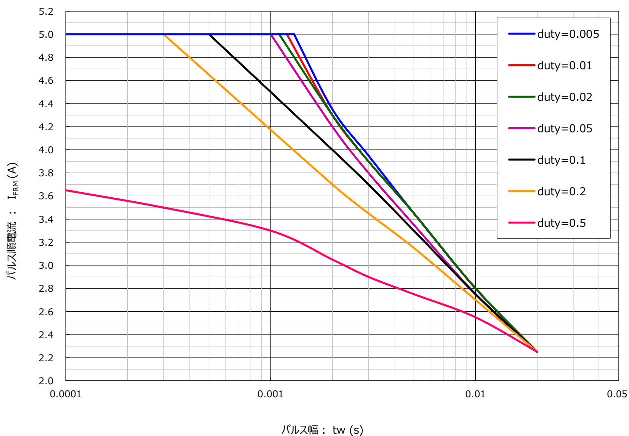
パルス順電流定格
