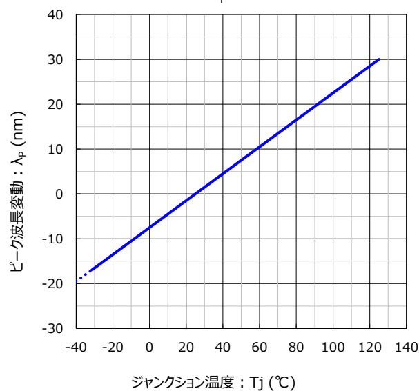
ジャンクション温度 vs. ピーク波長変動
