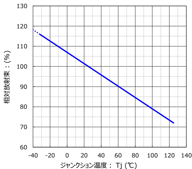
ジャンクション温度 vs. 相対放射束 特性
