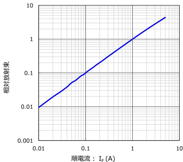
順電流 vs. 相対放射束 特性
