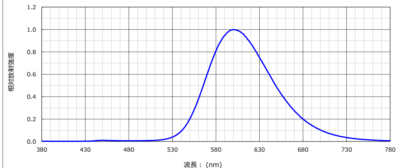
スペクトル分布特性 条件 : I_F = 140\text{mA} , T_a = 25^\circ\text{C}
