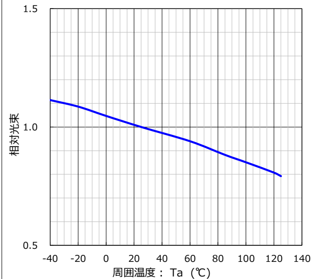
周囲温度 vs. 相対光束 特性
