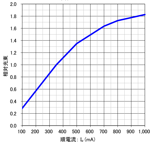
順電流 vs. 相対光束 特性
