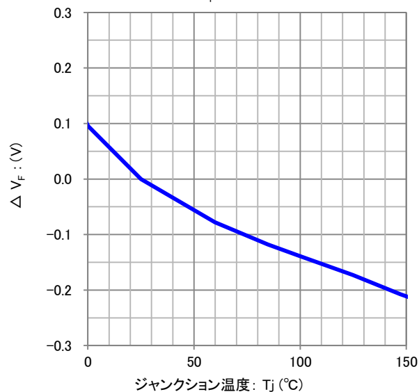
ジャンクション温度 vs. 順電圧 特性
