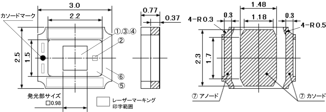
上面図
