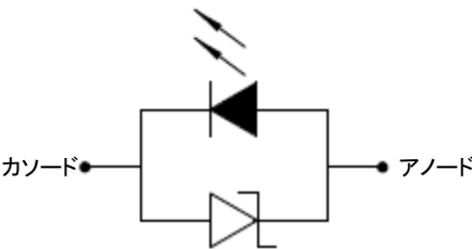
内部回路
