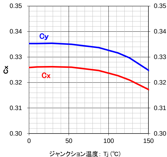
ジャンクション温度 vs. 色度 特性
