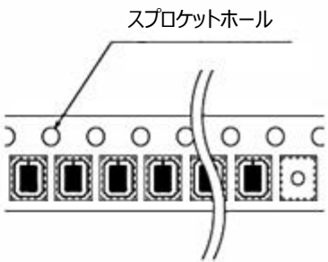
A部詳細-1
