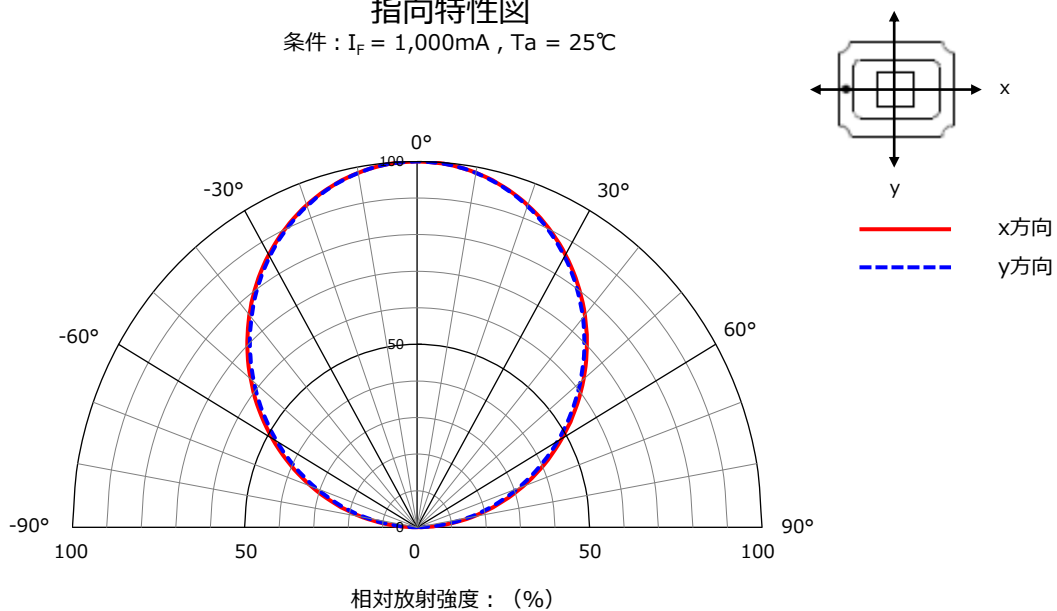
指向特性図
