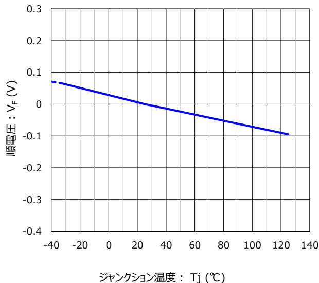
ジャンクション温度 vs. 順電圧 特性 条件 : I_F = 0.7\text{A}
