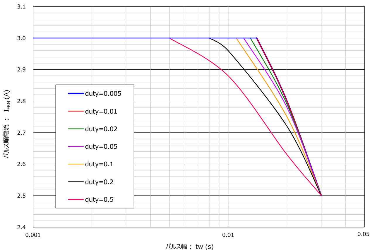
パルス順電流定格
