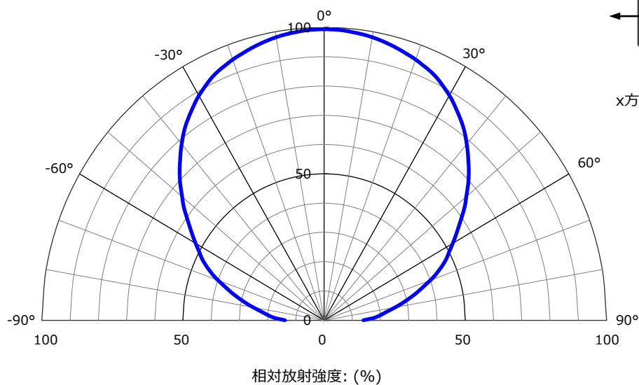
指向特性図
