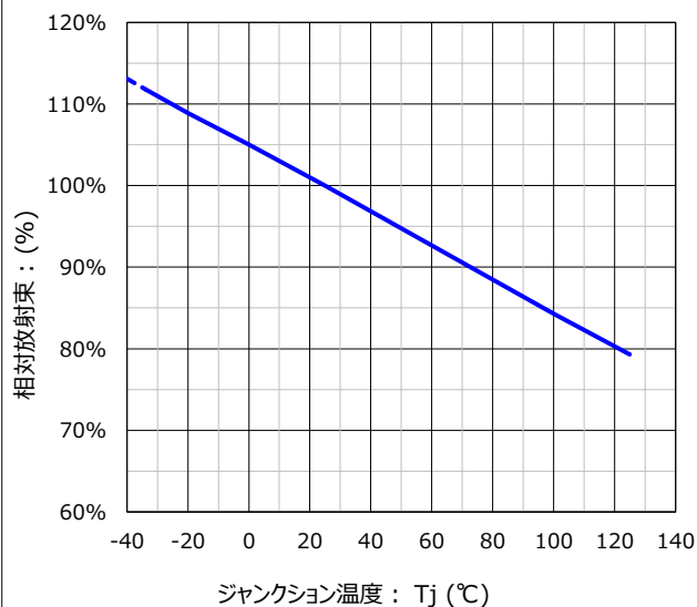
ジャンクション温度 vs. 相対放射束 特性 条件 : I_F = 0.7\text{A}
