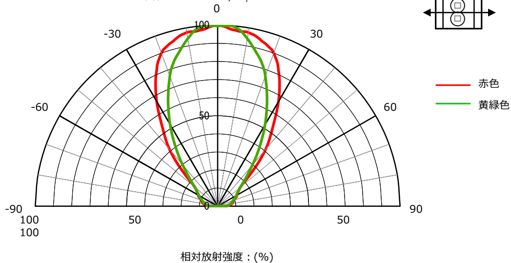
指向特性図
