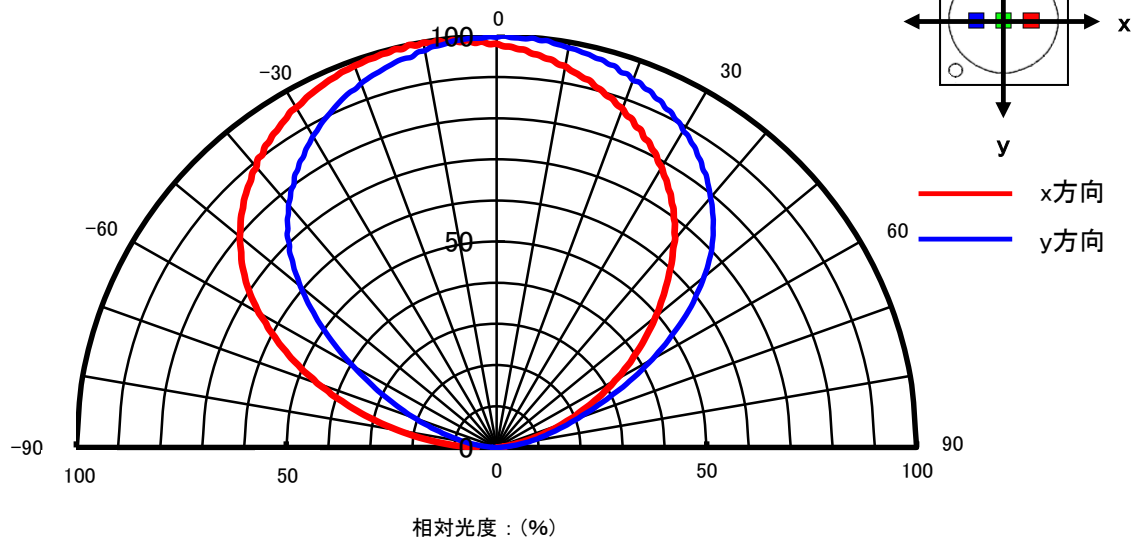
指向特性図
