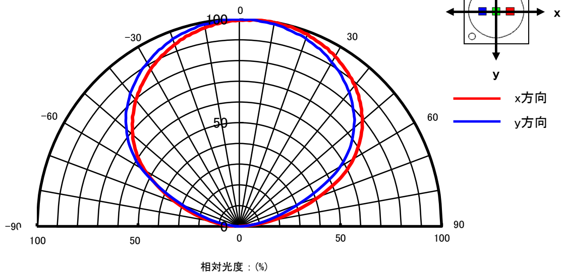
指向特性図
