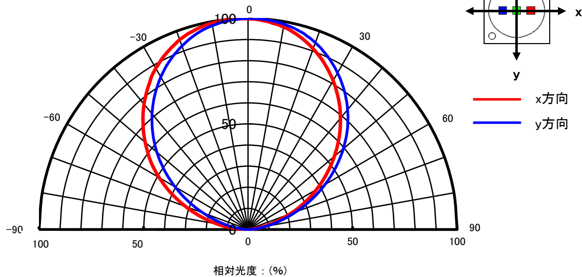
指向特性図
