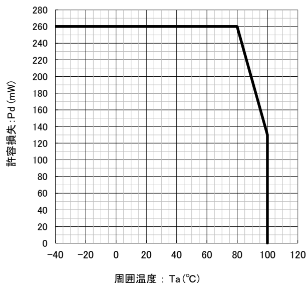
許容損失定格【緑色】
