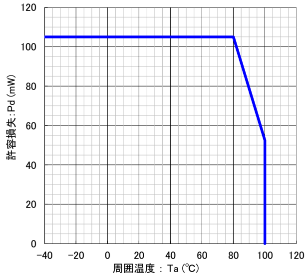
許容損失定格【青色】
