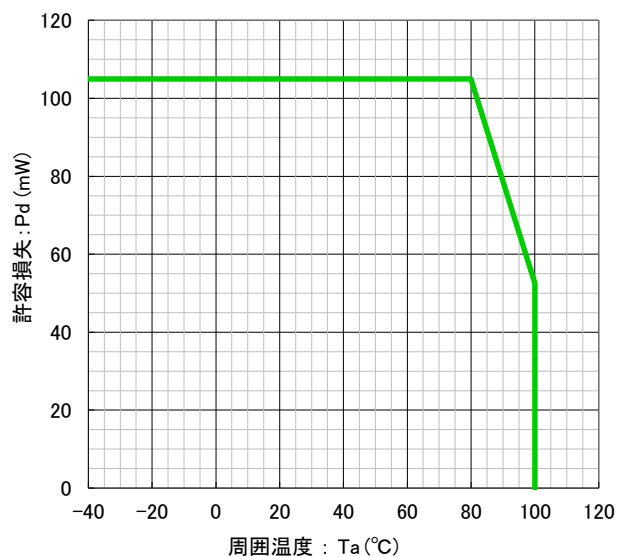
許容損失定格【緑色】
