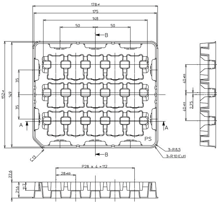
A-A 断面図
