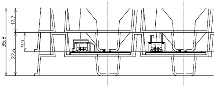
段積み形態図
