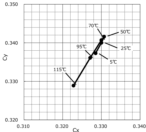
基板裏面温度 vs. 色度 特性
