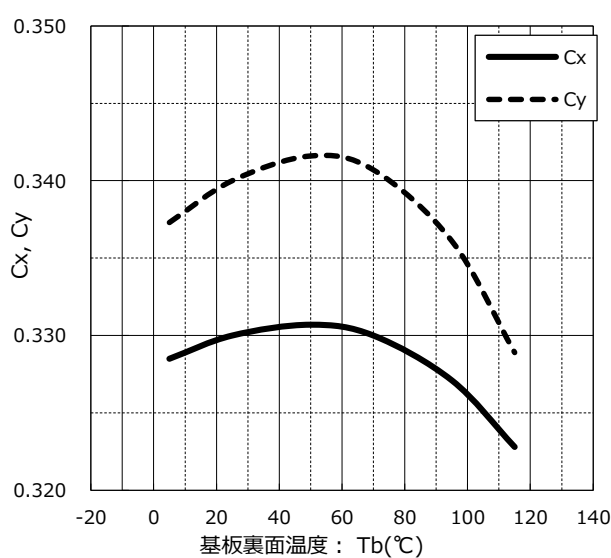
基板裏面温度 vs. 色度 特性
