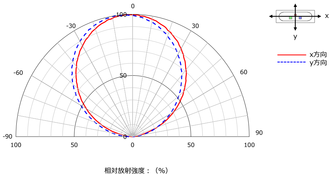
指向特性図
