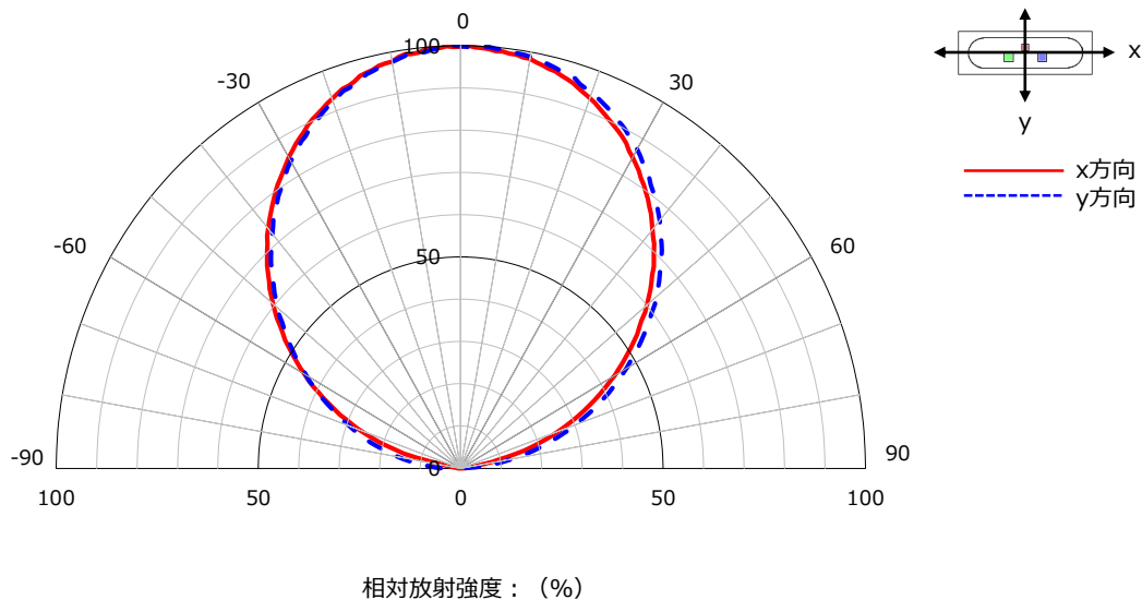
指向特性図
