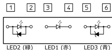
内部回路
