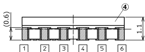
底面図
