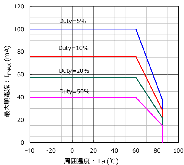
パルス順電流低減定格 繰り返し周波数: f \geq 50\text{Hz}
