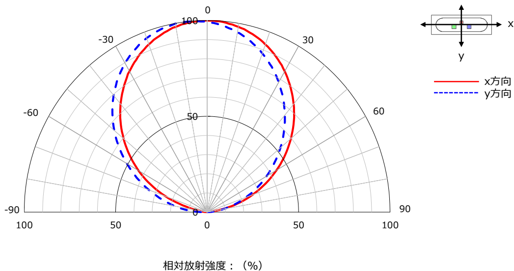
指向特性図 条件: I_F = 20\text{mA} , T_a = 25^\circ\text{C}
