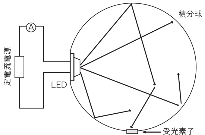
図2. 光束・放射束測定
