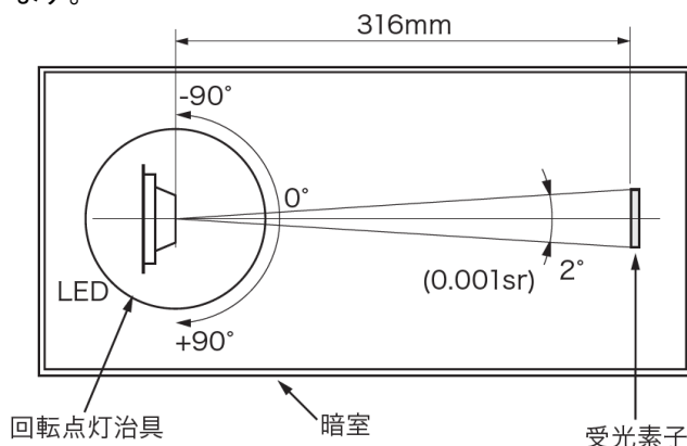
図5. 指向特性測定
