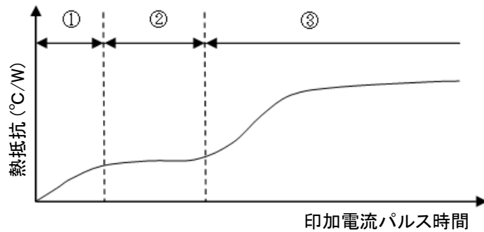
図11. 印可電流パルス時間と熱抵抗の特性
