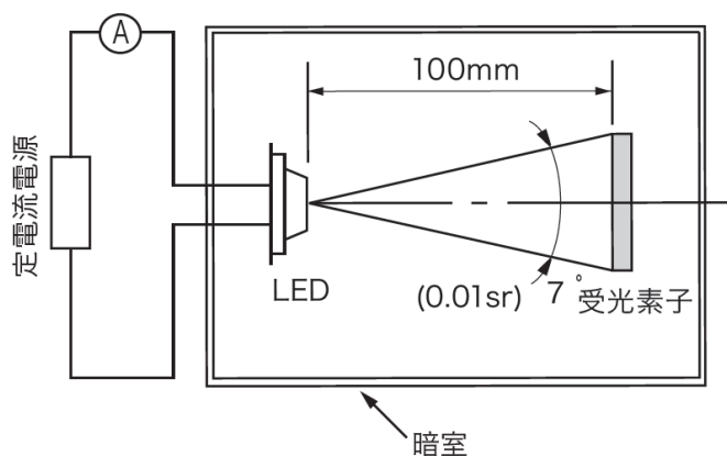
図3. 放射強度測定
