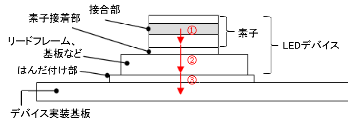
図12. 熱伝導経路
