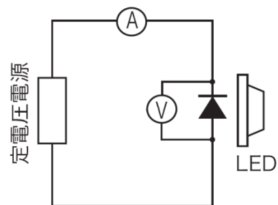
図9. 逆電流測定
