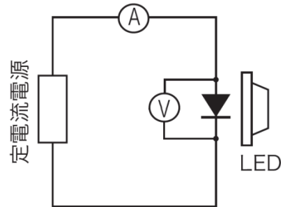
図8. 順電圧測定
