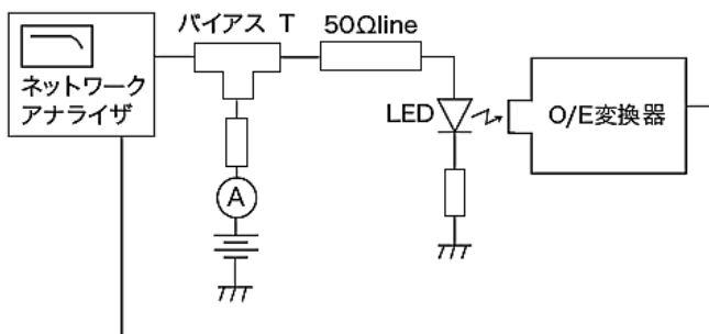
図7. 遮断周波数測定
