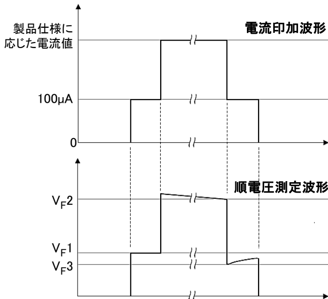
図10. 電流印可波形と順電圧測定波形の関係
