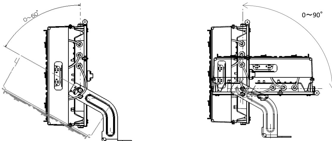
下向きアーム灯具の回転範囲 / Rotation range of downward arm lamp 上向きアーム灯具の回転範囲 / Rotation range of upper arm lamp
